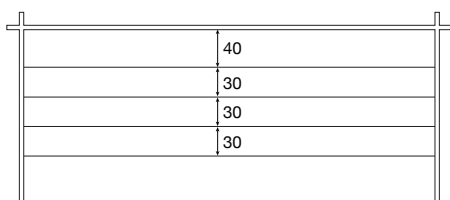
Structure 135 et 150
