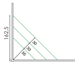
Structure 120 : 3 marches
