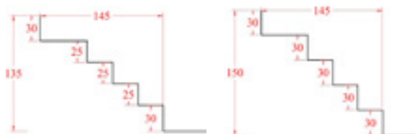
STRUCTURE 135 : 4 marches
